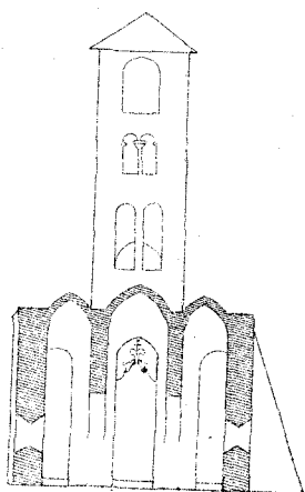
3 o Eglise de St Victor - Coupe transversale
