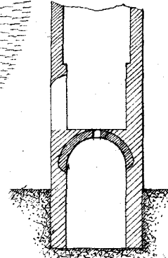
Coupe de la tour des prisons
