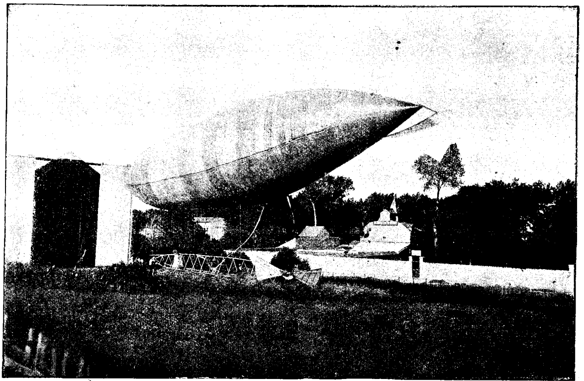
LE « SANTOS-DUMONT » VU DE L'ARRIÈRE
