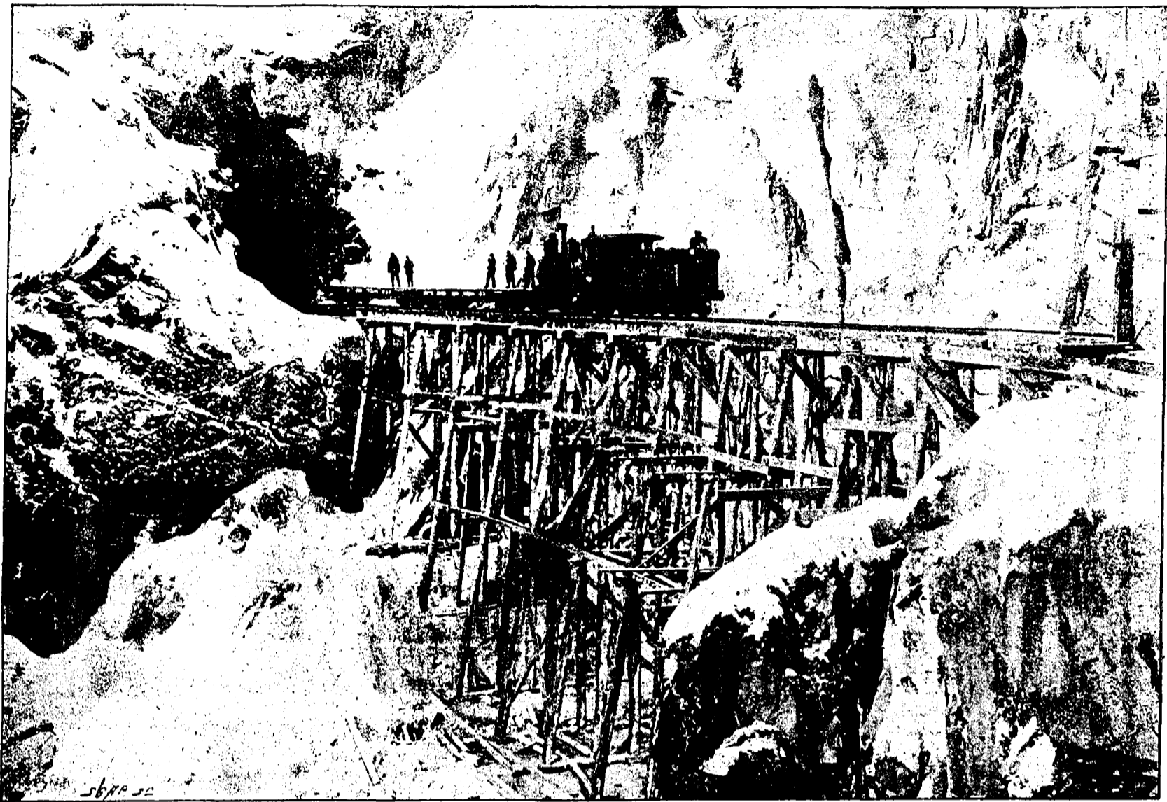
Le Tunnel du Chemin de fer de la White-Pass à Skagway (Alaska).
