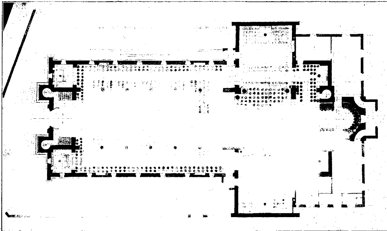
ÉGLISE SAINT-AUGUSTIN A LYON. — PLAN. — ARCHITECTE, M. A. CHOMEL
